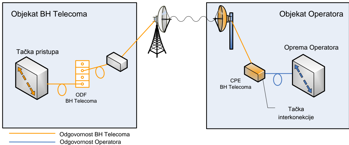
Slika 3: Šematski prikaz realizacije interkonekcije na strani Operatora putem optičkog povezivanja ili RR veze
